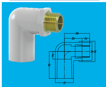
Co 90° / 90° Elbow
